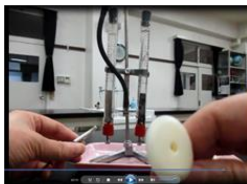
図2 燃料電池の仕組みを確認する実験
