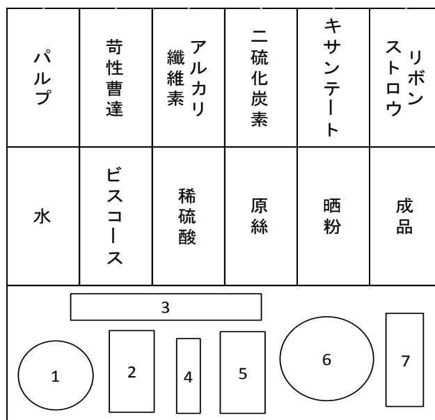
図 14 図 13 の原材料、中間品、製品の配置 (下段の番号は 図 16 を参照)
