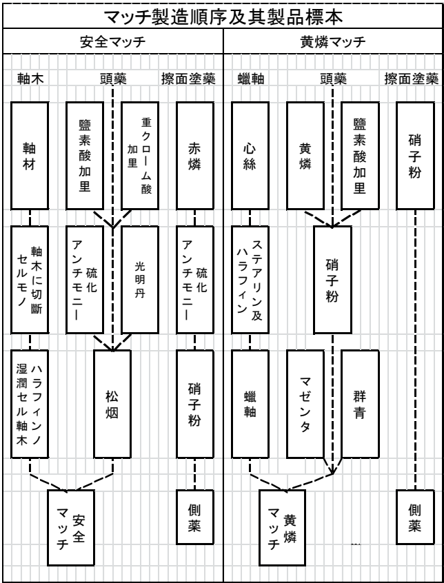
図 2 図 1 の原材料、中間品、製品の配置
