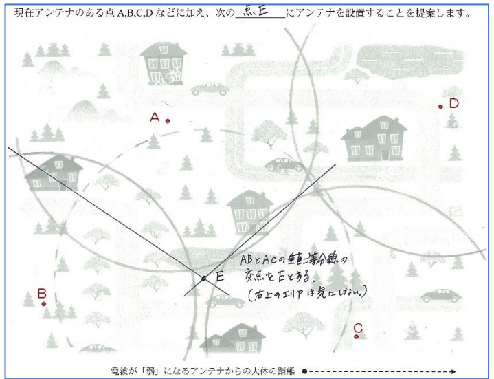
図8 垂直二等分線の交点に1つめを決める。
