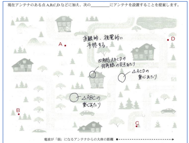
図2 直観的に予想する。
