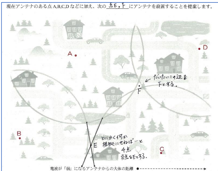
図7 「この辺」に論理らしきものを付随させて決める。
