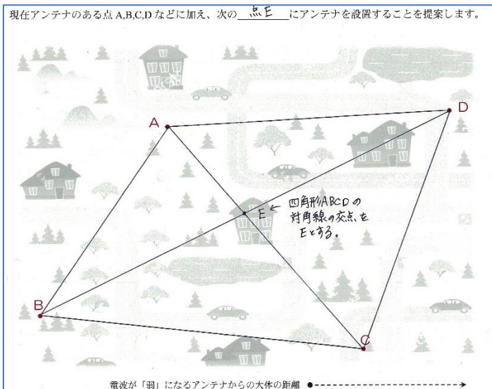
図3 四角形の対角線の交点をEとする。
