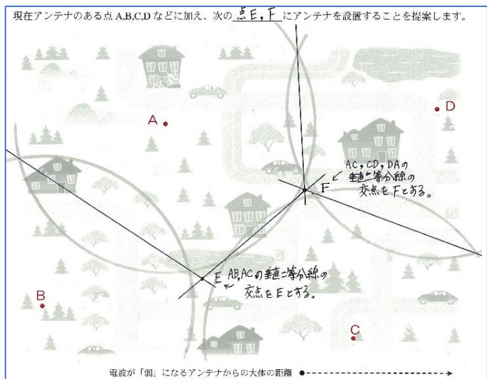
図9 別の垂直二等分線の交点に2つ目も決める。
