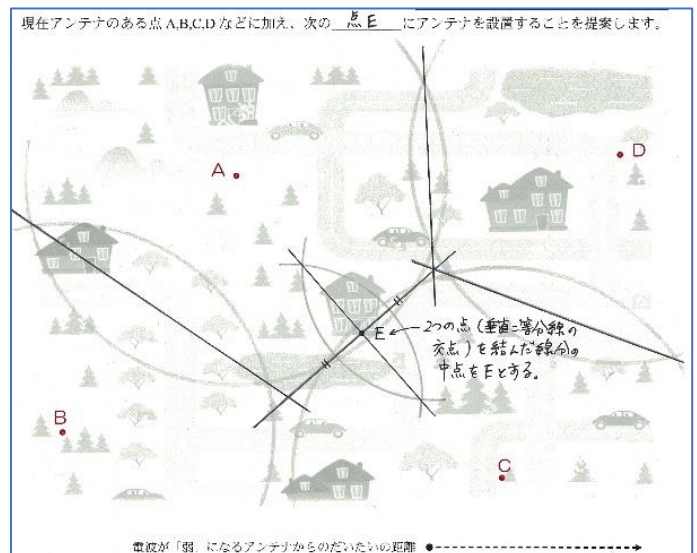
図11 2点に決めるために、間をとる。
