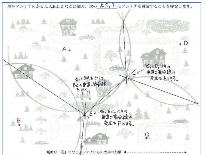
図10 BCの垂直二等分線を新たに書き加える。
